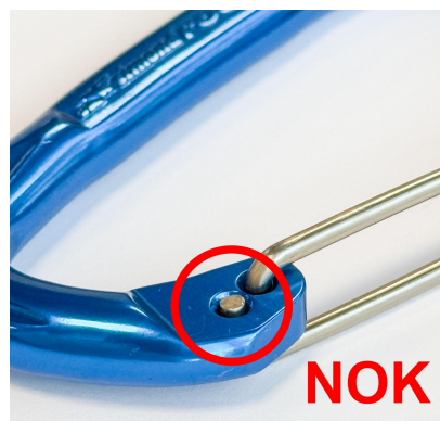
Klinkverbinding niet OK, plat uiteinde
