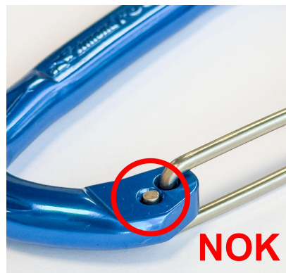
Nituire NOK, capăt plat
