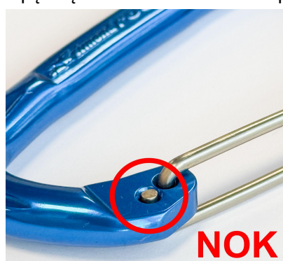
Nitowanie nieprawidłowe, płaski koniec
