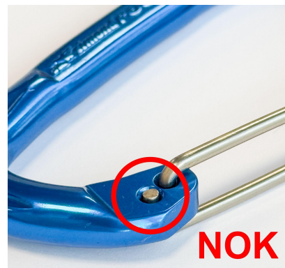
Rivettatura NOK, estremità piatta
