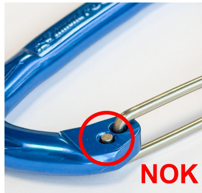
Remachado NOK, extremo plano
