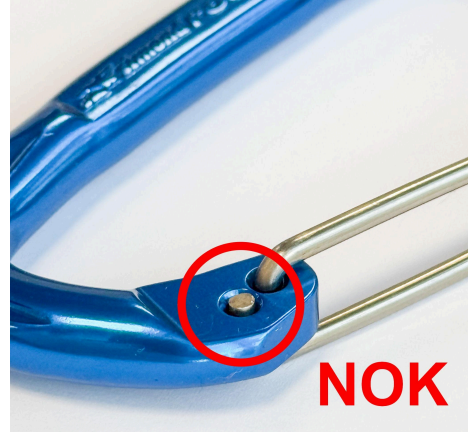
Fotoğraf 2: Perçinleme hatalı (NOK), düz
