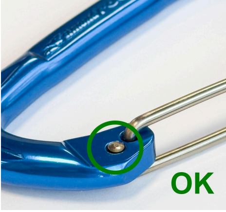
Fotoğraf 1: Perçinleme uygun (OK), yuvarlak uçlu; uçlu, mantar şeklinde.
